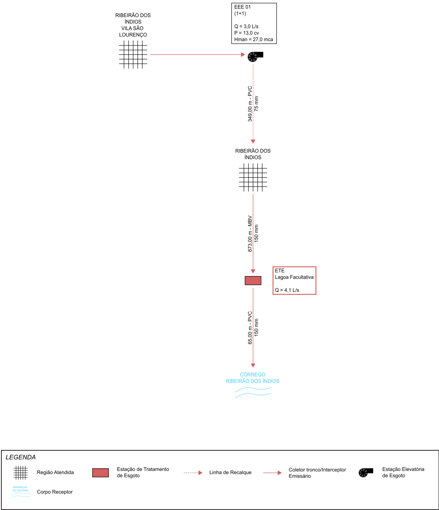
Figura 4.2 – Croqui do Sistema de Esgotamento Sanitário da Sede de Ribeirão dos Índios
